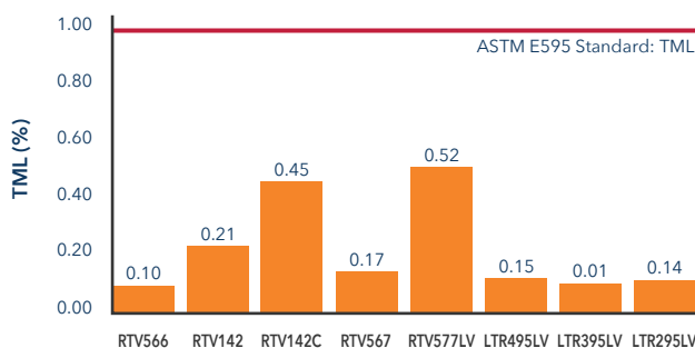
ASTM E595 Results: TML (≤1.00%)
